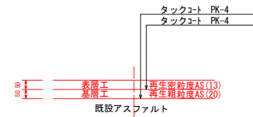
施工要領図
